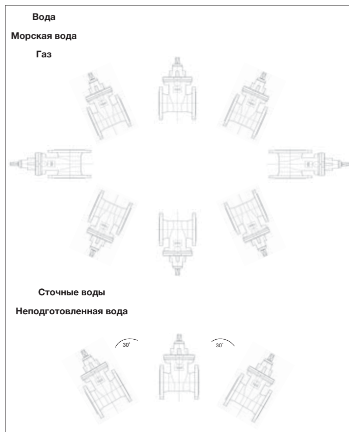
Рис. 5: Положение задвижки при установке
