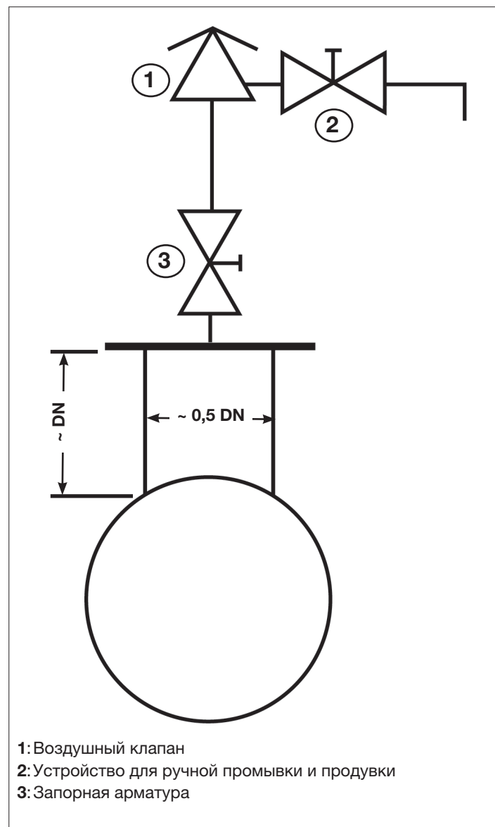
Рис. 7: Трубопровод < DN 600
