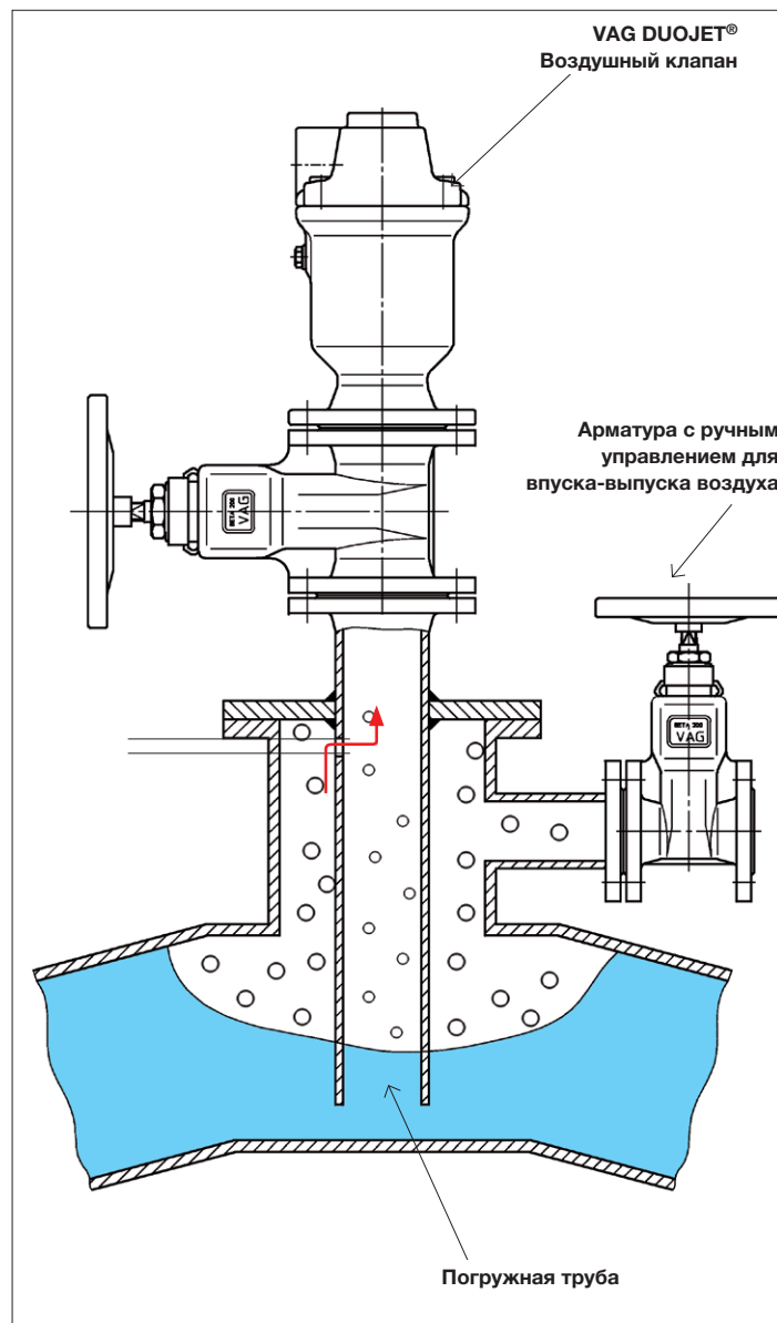
Рис. 9: Купол с погружной трубой
