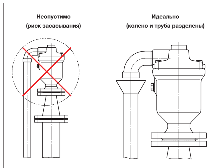
Рис. 13: Установка при сбросе разбрызгиваемой воды
