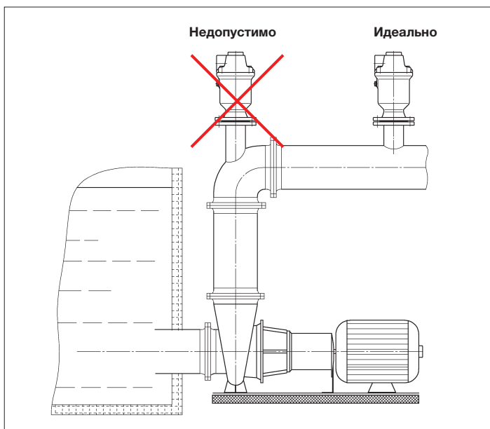
Рис. 11: Установка после насоса
