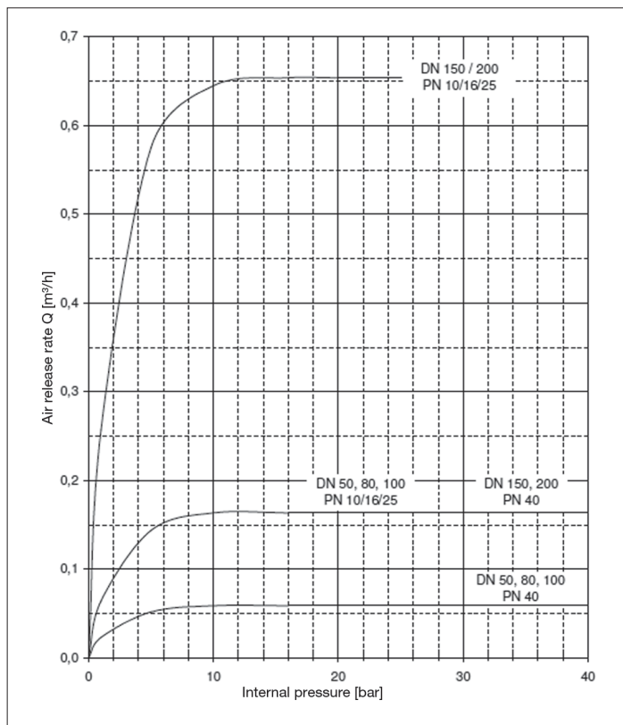
Рис. 6: Выпуск воздуха - малое сечение
