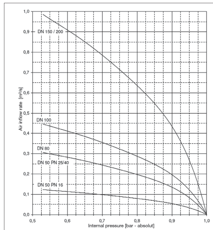
Рис. 4: Впуск воздуха - большое сечение
