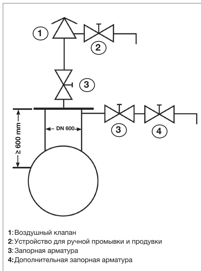
Рис. 8: Трубопровод \geq DN 600
