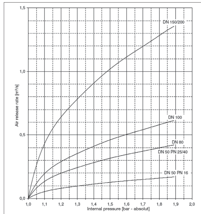
Рис. 5: Выпуск воздуха - большое сечение
