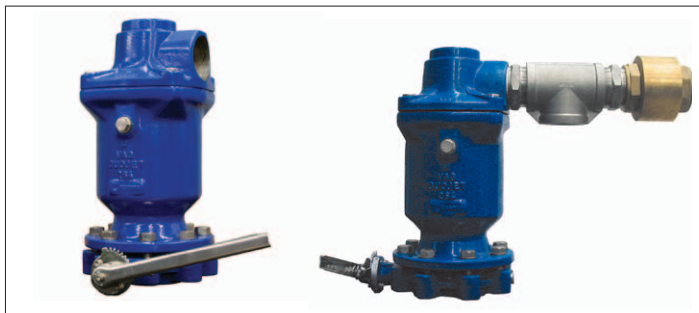
Рис. 3: Варианты VAG DUOJET®-S и VAG DUOJET® Anti-Surge
