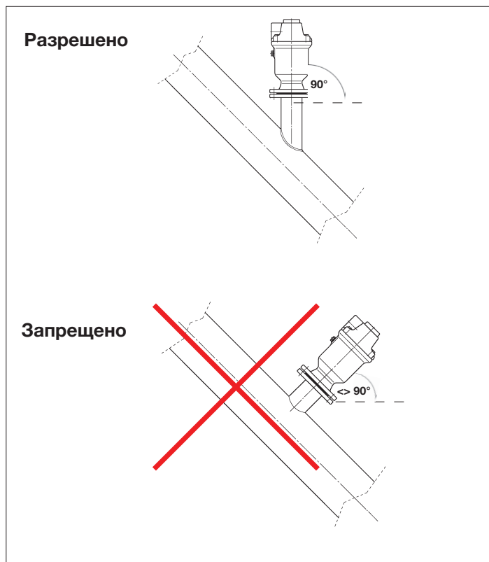
Рис. 10: Положение при установке
