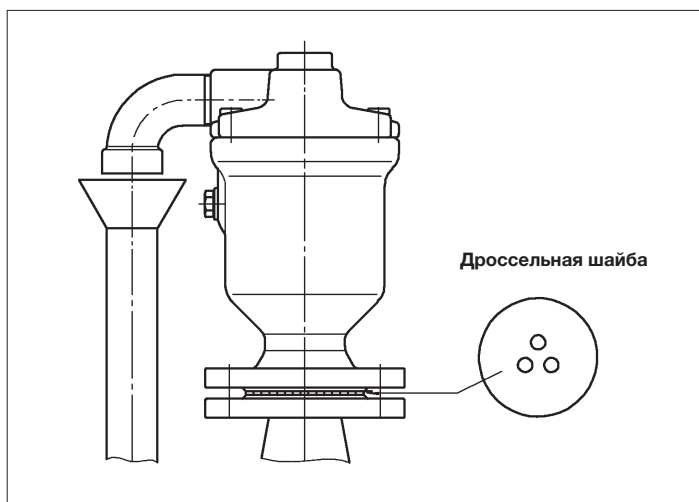
Рис. 12: Установка на подъёмном трубопроводе
